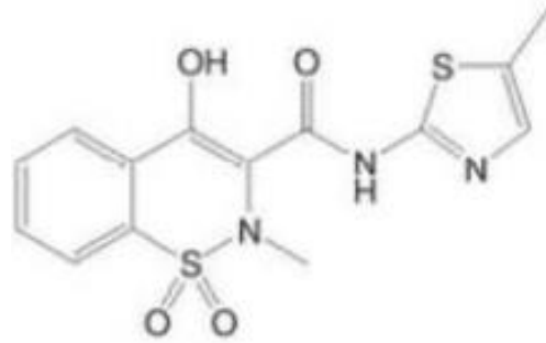
Meloxicam
