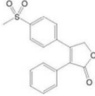
Rofecoxib
