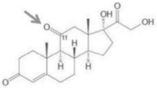
Cortisone
