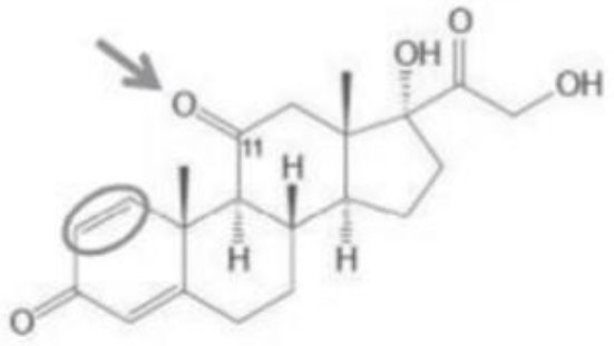
Prednisone
