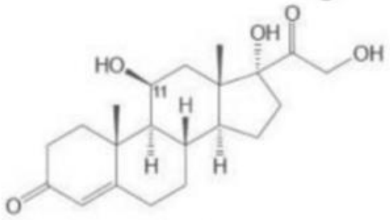
Cortisol
