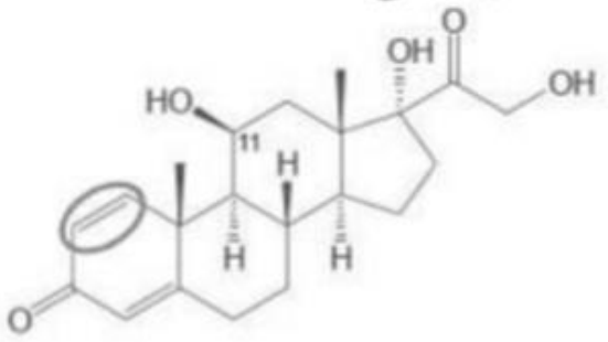
Prednisolone
